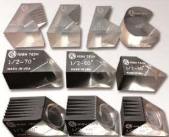
Cuñas acrílicas Quick Change 45°, 60°, 70° para Transductores de 1/2", 3/8", 1/4"
