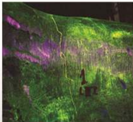
Inspección por Partículas Magnéticas vía Húmeda
